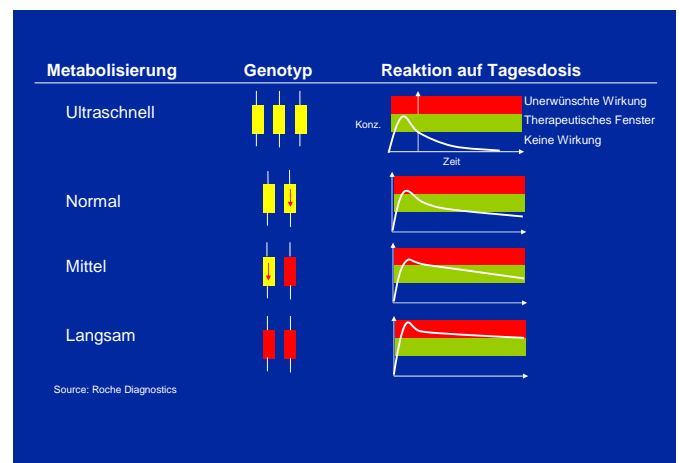
Abbildung 2: Einfluss des CYP450 -Genotyps auf den Medikamentenmetabolismus
